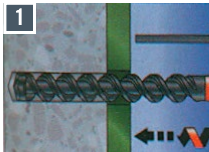
1. Bohrloch erstellen / Drill hole
