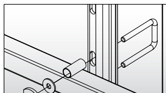
H-50 Halterung auf Sprosse H-50 rung assembly set
