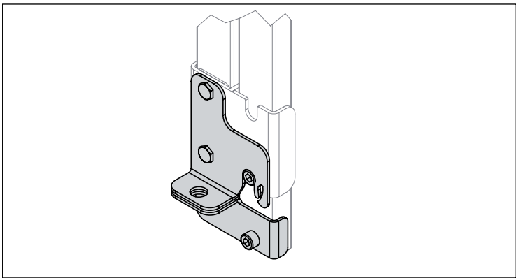
Erweiterung um Rastfunktion und Schlosslasche zur zusätzlichen Montage Additional part fits to connector to provide locking function and eyelet for padlock
